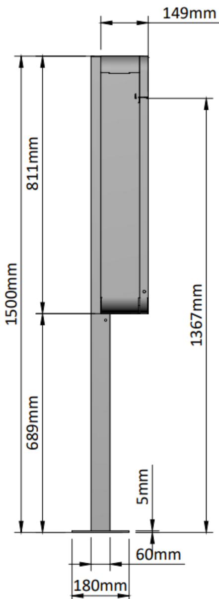
Abbildung seitlich mit Abmessungen bei Montage der Ladeeinrichtung mit LADE Standfuß
